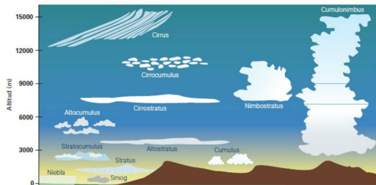
Vista de los diferentes géneros de nubes y los niveles aproximados que ocupan
